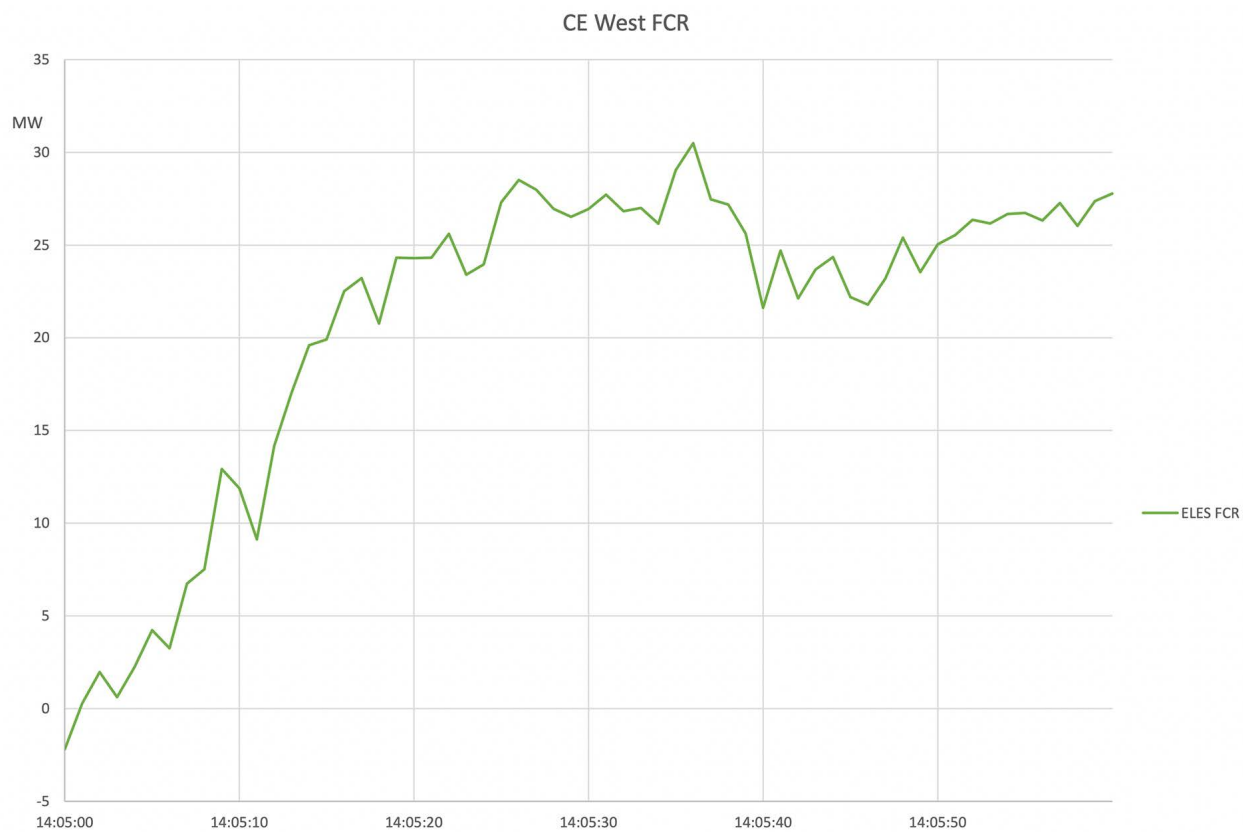
Figure A2-13: ELES FCR
